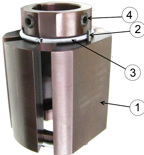
Parti del gruppo manicotto 514-9B
